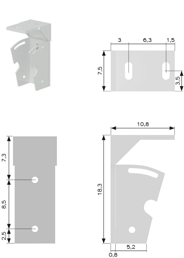
STAFFA A SOFFITTO
