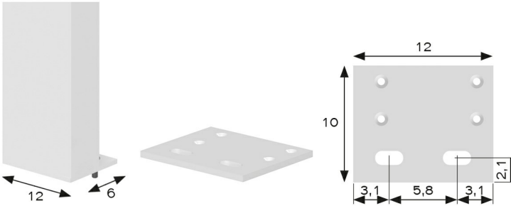
GAMBA SUPPLEMENTARE COMPLETA CON PIEDE FISSO (DI SERIE)
