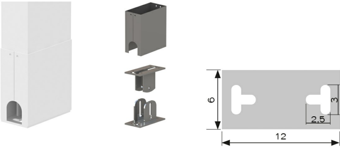
GAMBA SUPPLEMENTARE COMPLETA CON PIEDE REGOLABILE (A RICHIESTA)
